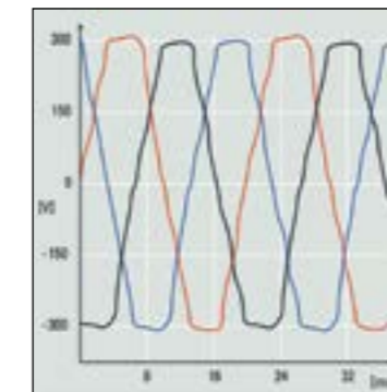
Målingene viser tydelig forvrenging i nettspenningens bølgeform som følge av forstyrrelser fra ikke-lineære belastninger.
